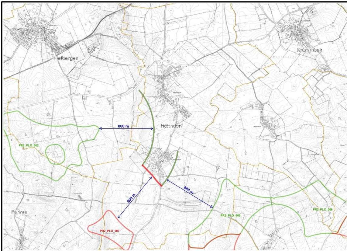
Abbildung 14: Abstände der Vorrangflächen und abgelehnten Potentialflächen zur Ortslage von Höndorf
