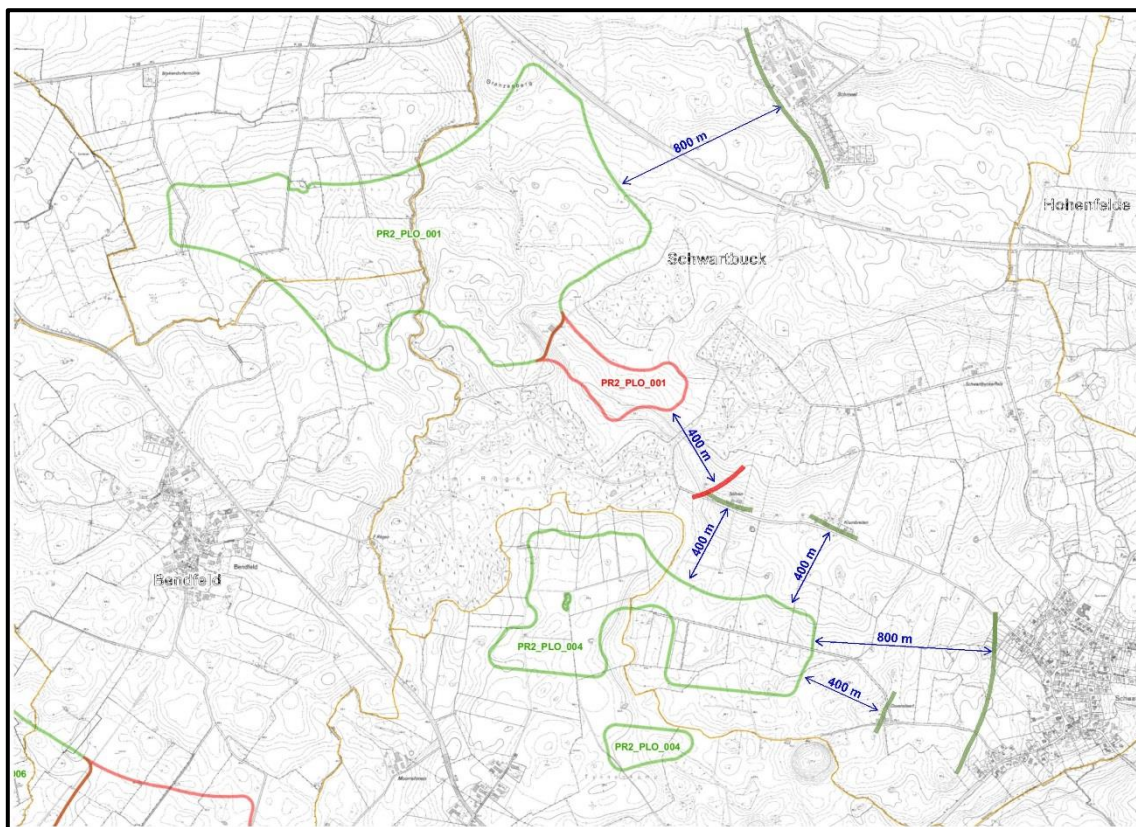
Abbildung 12: Abstände der Vorrangflächen und abgelehnten Potentialflächen zur Ortslage von Schwarzbuck
